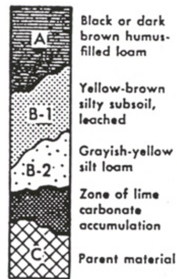
Chernozem
