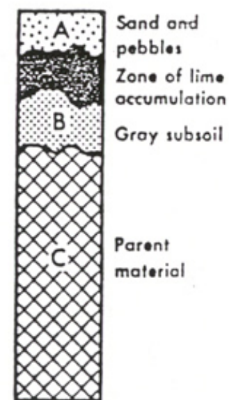
Sierozem
