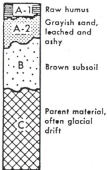
Podzol
