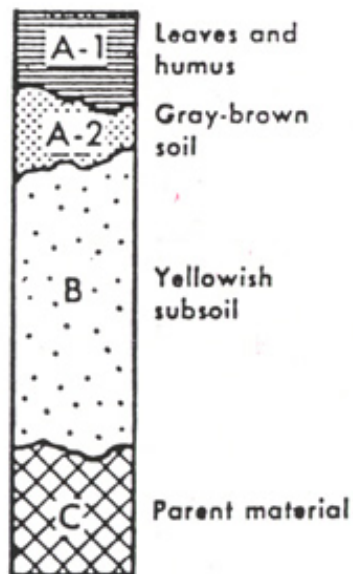
Grey-Brown Podzol
