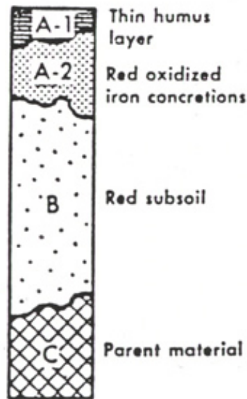
Latosol
